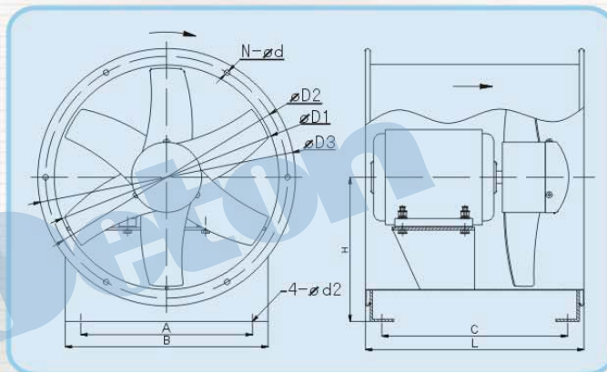
T40A式轴流风机外形尺寸表
